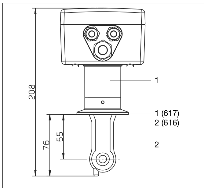
Исполнение с подключением к процессу 616 = Clamp 2 1/2" 617 = Clamp 2 1/2" и типовым дополнением 757 и 941 (крепежная скоба не входит в комплект поставки)
