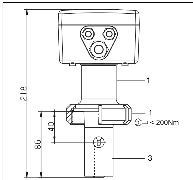
Исполнение с подключением к процессу 690 = SMS 2" ( \hookrightarrow < 200Nm) и типовым дополнением 768
