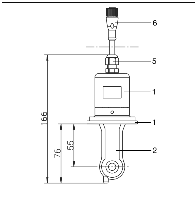
Раздельное исполнение с подключением к процессу 690 = SMS 2" ( \hookrightarrow < 200Nm) и типовым дополнением 767 и 941 (накидная гайка не входит в комплект поставки)
