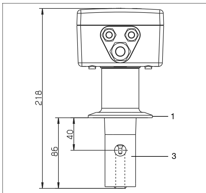
Исполнение с подключением к процессу 617 = Clamp 2 1/2" и типовым дополнением 768 (крепежная скоба не входит в комплект поставки)
