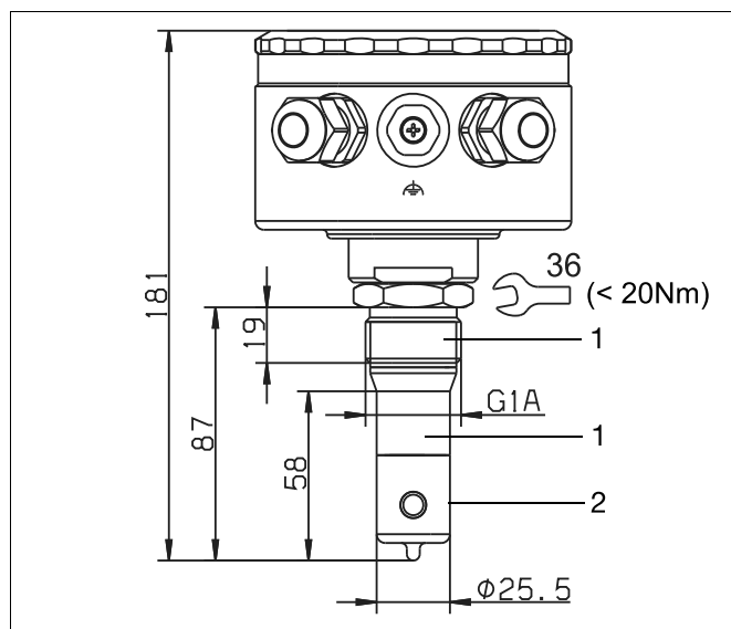
Исполнение с подключением к процессу 956 = прижимное соединение G 1" ( \hookrightarrow < 20Nm) EL = 87 мм
