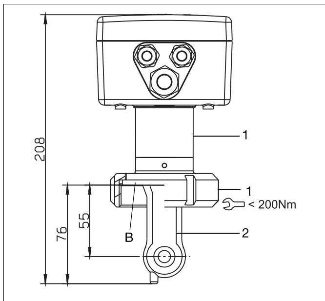
Исполнение с подключением к процессу 690 = SMS 2" ( \hookrightarrow < 200Nm) и типовым дополнением 767 и 941
