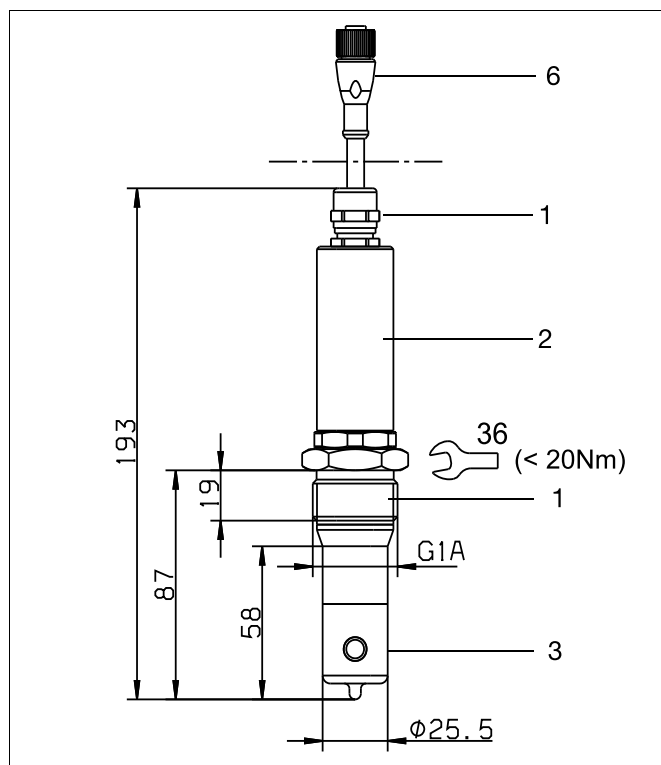
Раздельное исполнение с подключением к процессу 956 = прижимное соединение G 1" ( \hookrightarrow < 20Nm) EL = 87 мм И типовым дополнением 767
