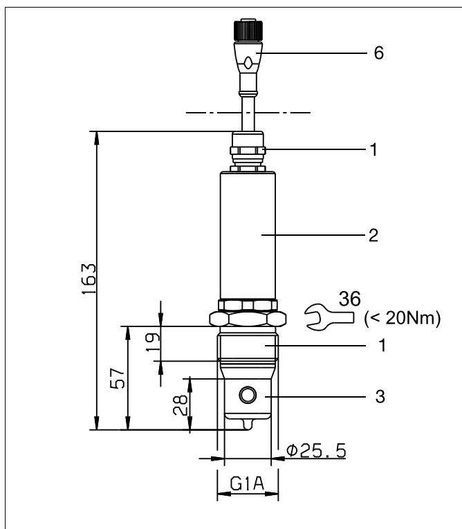
Раздельное исполнение с подключением к процессу 955 = прижимное соединение G 1" ( \hookrightarrow < 20Nm) EL = 57 мм И типовым дополнением 767
