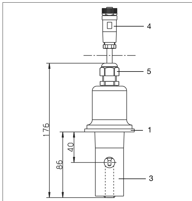
Раздельное исполнение с подключением к процессу 690 = SMS 2" ( \hookrightarrow < 200Nm) и типовым дополнением 768 (накидная гайка не входит в комплект поставки)
