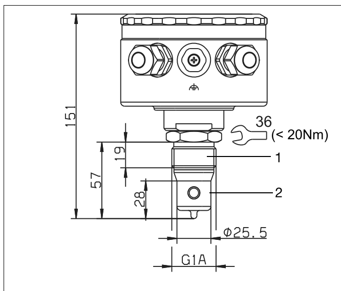
Исполнение с подключением к процессу 955 = прижимное соединение G 1" ( \hookrightarrow < 20Nm) EL = 57 мм
